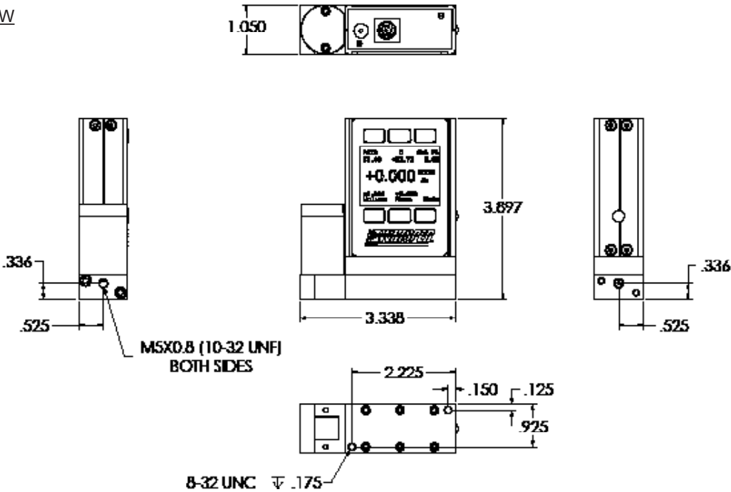
MCW 0.5 sccm till 20 sccm ungefärlig transportvikt: 499 gram
