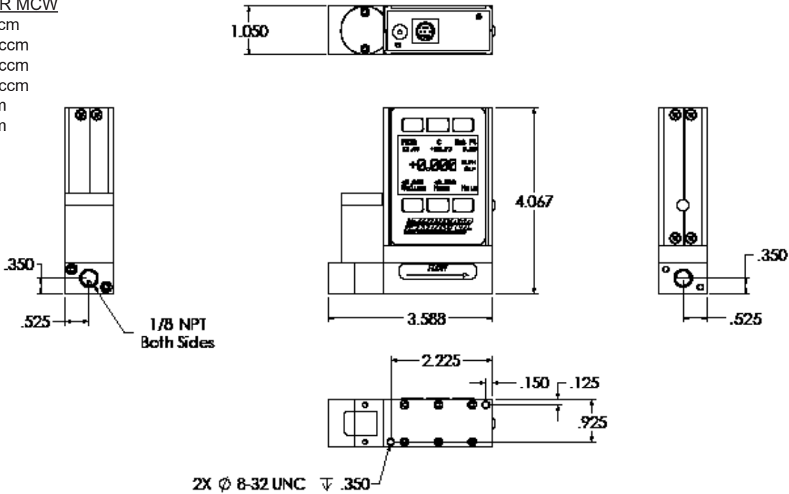
MCW 50 sccm till 2 slpm ungefärlig vikt: 544 gram
