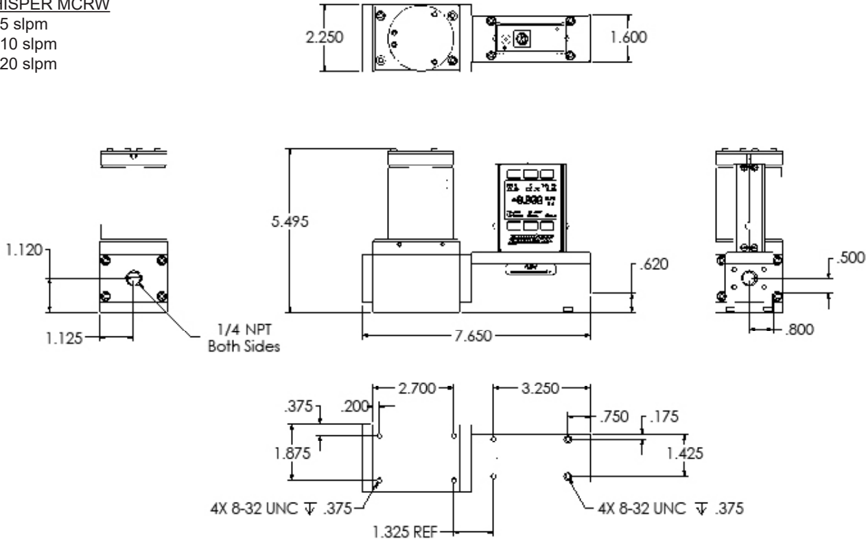
MCRW 50 slpm till 20 slpm ungefärlig vikt: 2903 gram
